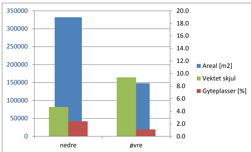
Figur 31: En sammenligning av vanndekt areal (blått), skjultilgang (grønt) og gytearealandel (rødt) sett for strekingen nedenfor og ovenfor Helvetesfossen.
