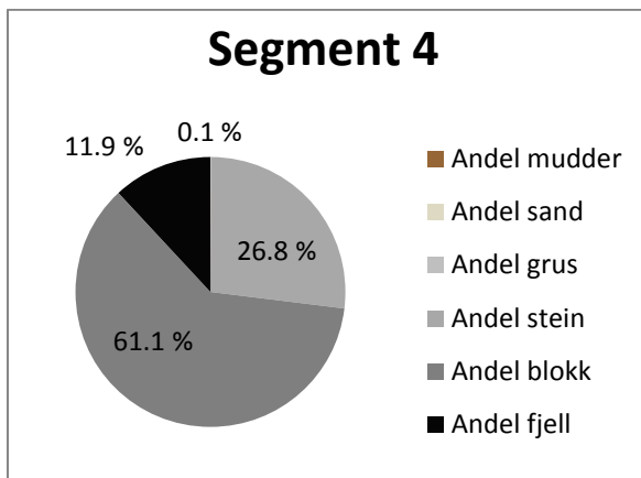
Figur 18: Blokk og rullestein dominerer substratet ovenfor Helvetesfossen.
