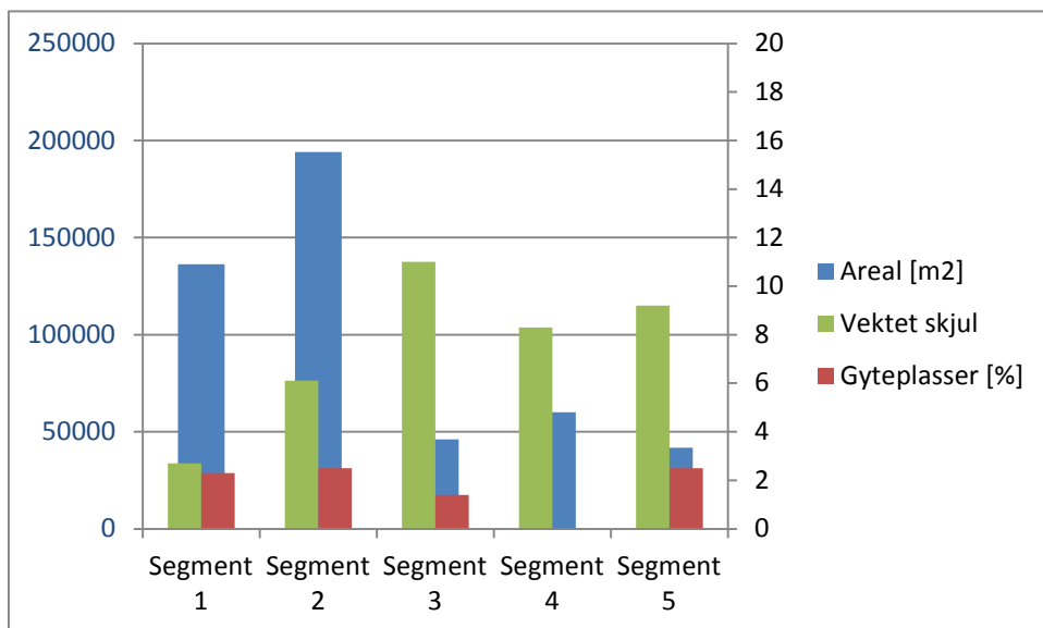
Figur 30: En sammenligning av vanndekt areal (blått), skjultilgang (grønt) og gytearealandel (rødt) per segment, ved vannføring på ca. 20 m 3 /s ndf. Helvetesfossen og 1,3 m 3 /s ovenfor.
