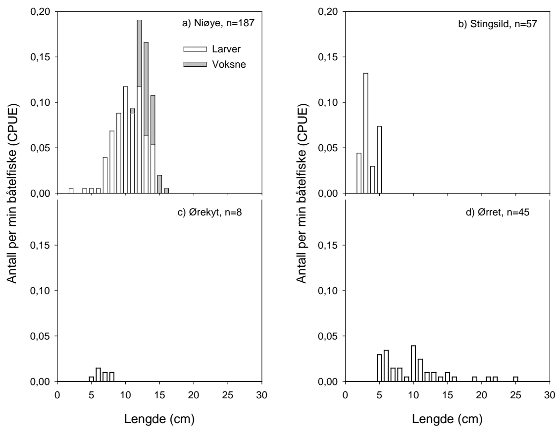
Figur 4.10. Lengdefordeling av a) niøye, b) stingsild, c) ørekyt og d) ørret fanget med elbåt på deltaet og i Tokkeåi i 2012.
